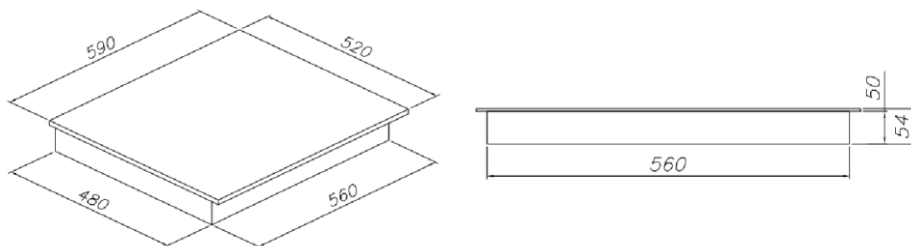
Διαστάσεις προϊόντος
