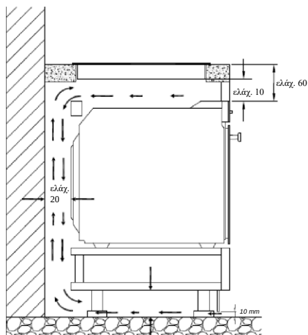
Βάση φούρνου
