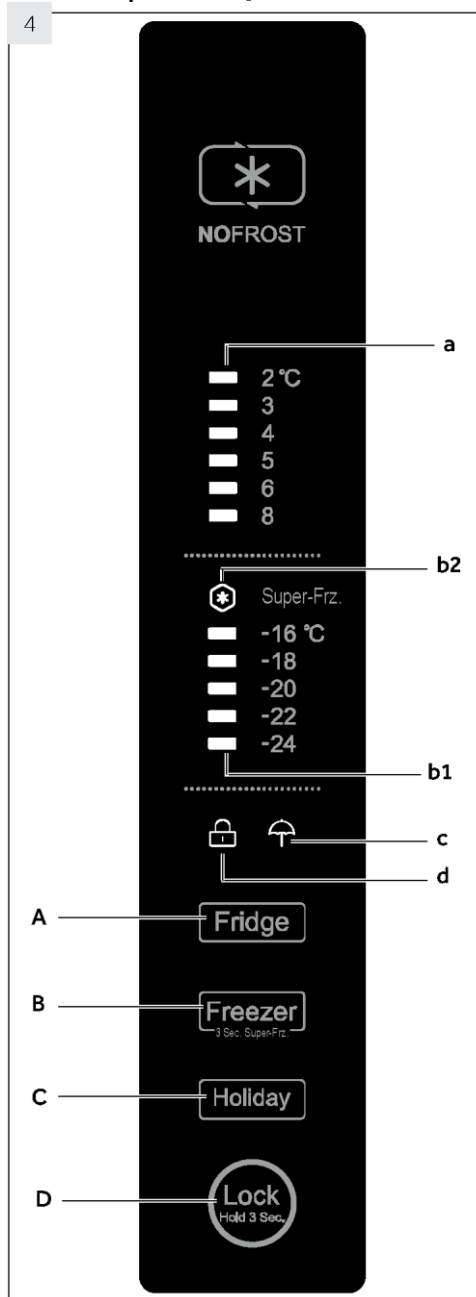
Vadības panelis (4. att.)
