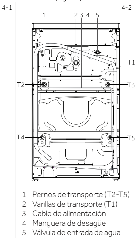
Parte trasera (Fig. 4-2):
