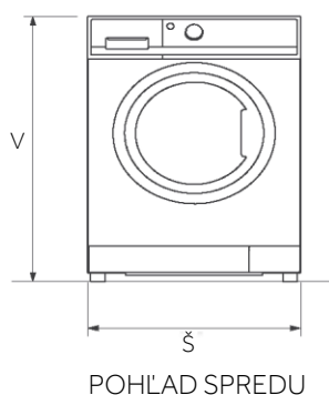
POHĽAD SPREDU
