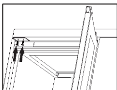
Držiak v tvare I
