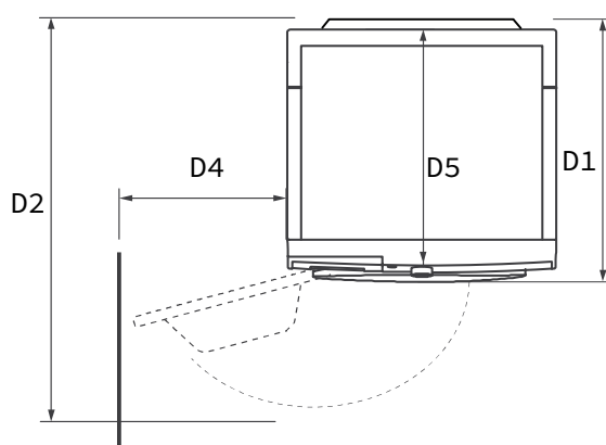
PARETE VISTA DALL'ALTO
