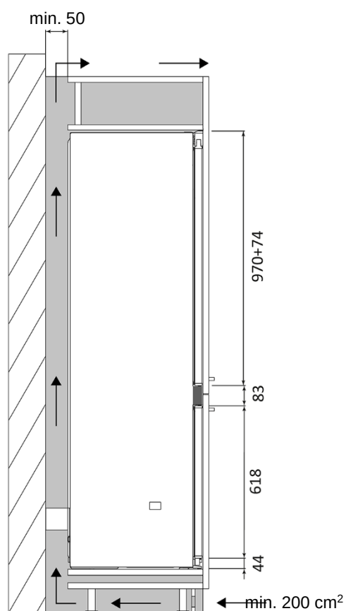
Przekrój boczny
