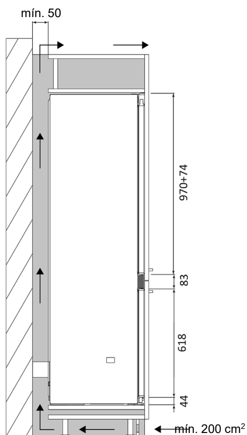
Sección lateral
