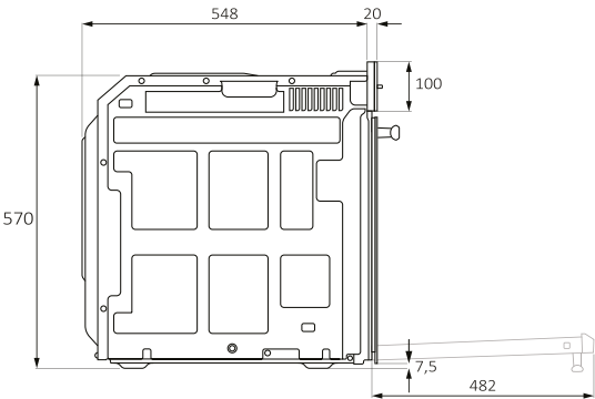
Külgvaade
