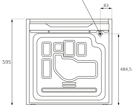
Achteraanzicht
