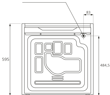
Widok tylny
