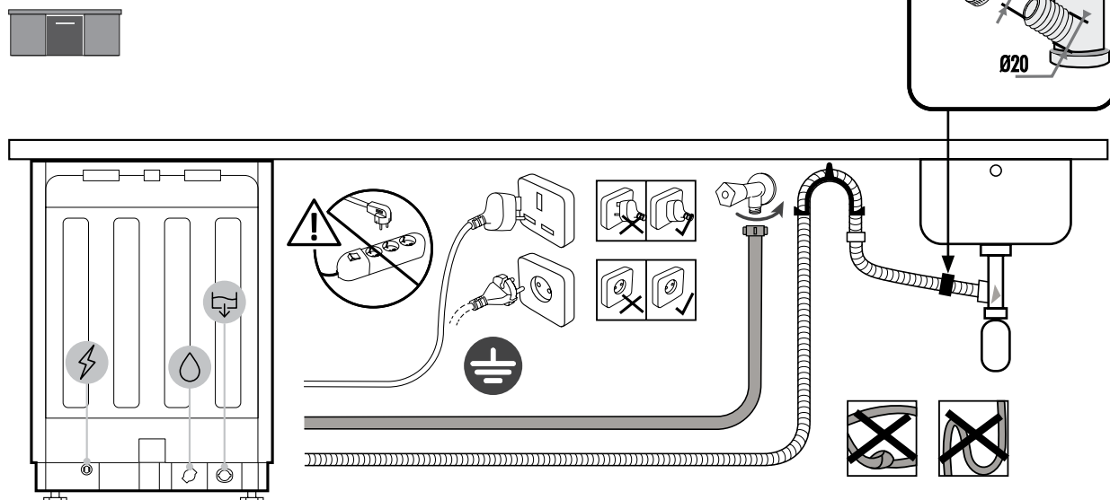
Esquema de instalação padrão
