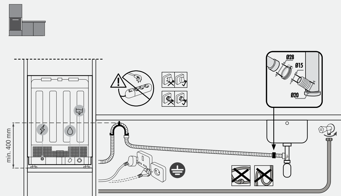
Esquema de instalação em coluna
