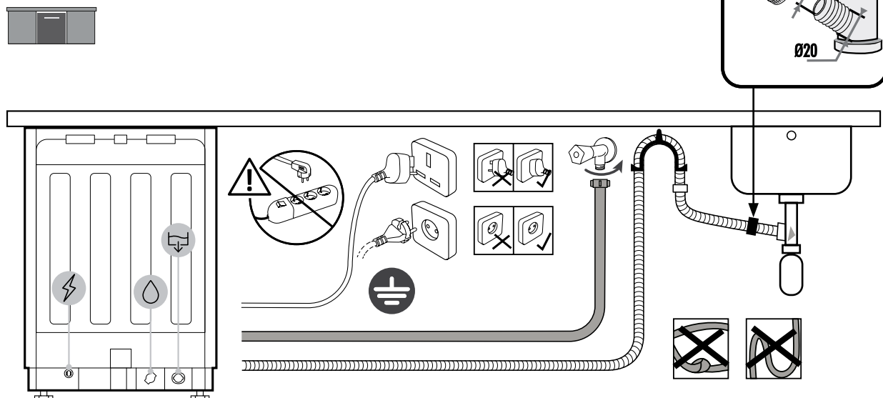
Стандартна монтажна схема
