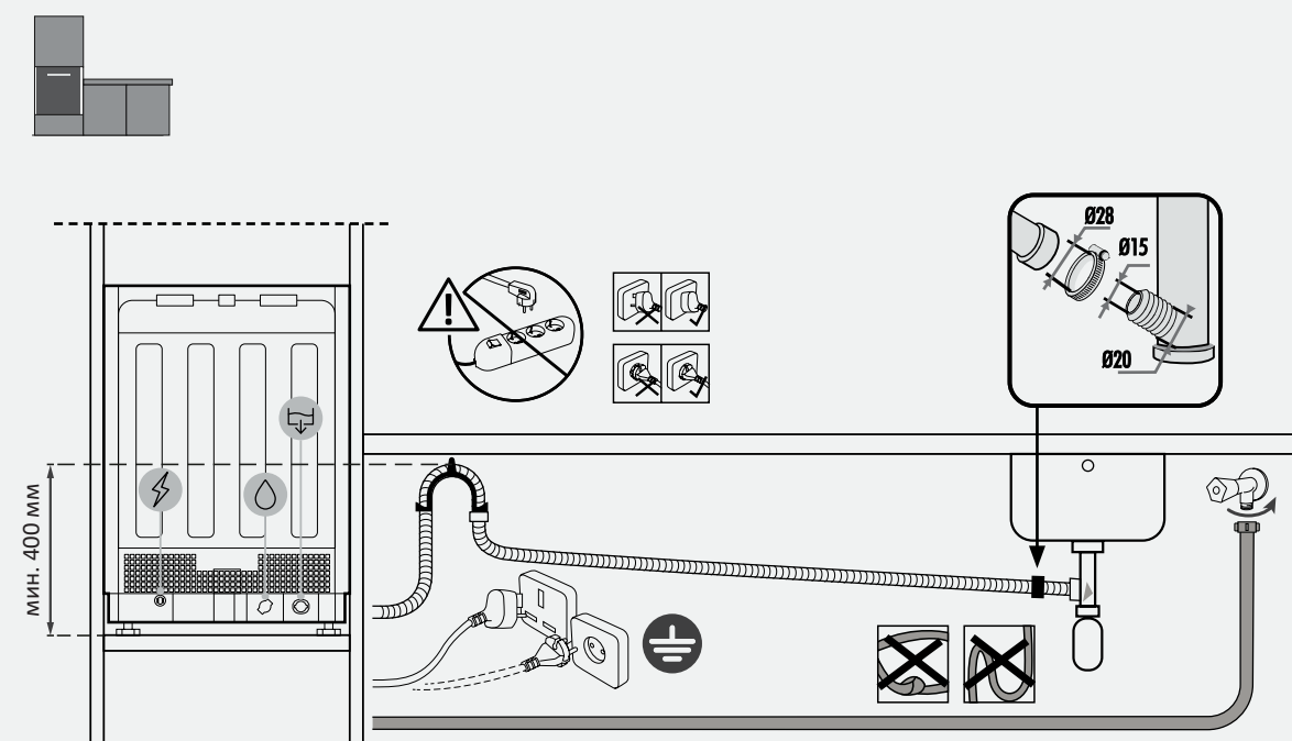
Схема за монтаж на колона
