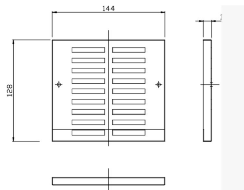
Detalhe da altura da grade
