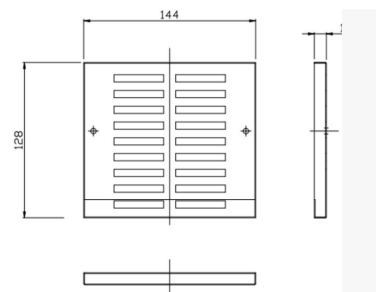
Détail de la hauteur de la grille
