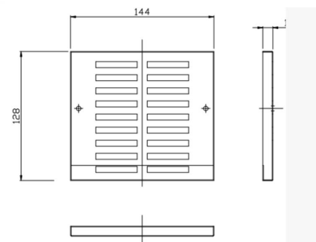
Dettaglio altezza griglia
