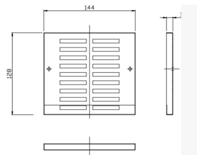
Detalle de altura de cuadrícula
