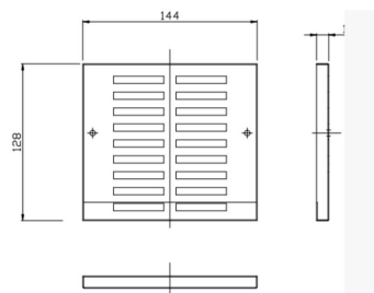
Szczegóły wysokości siatki
