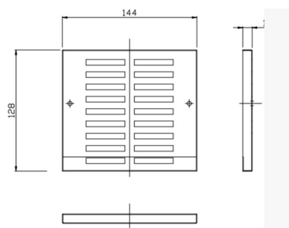
Detail výšky mřížky
