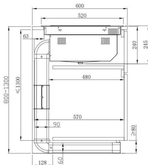
Filtreringsversion
