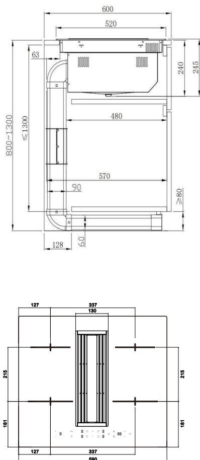
Version filtrante
