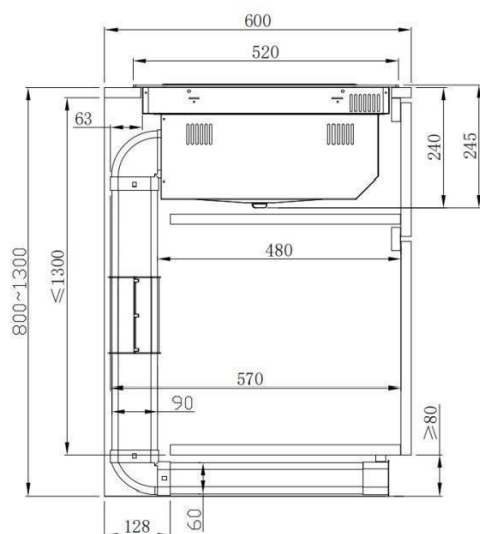
Filtrerande version
