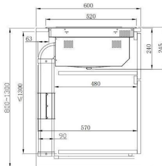
Udsugningsversion
