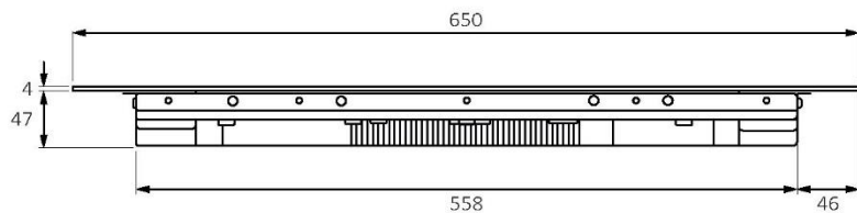
Vooraanzicht
