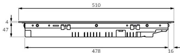
Vue latérale
