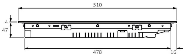
Seitenansicht
