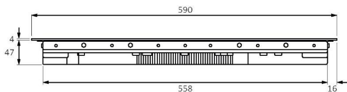
Vooraanzicht
