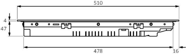
Vista lateral
