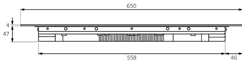
Vue frontale
