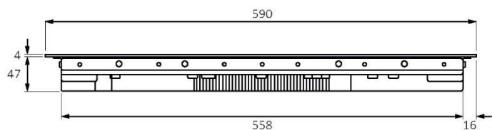
Vista anteriore
