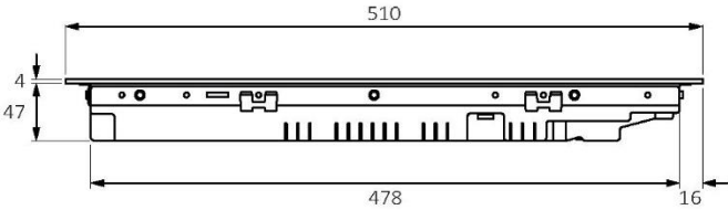
Vista lateral
