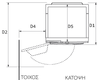
ΤΟΙΧΟΣ
