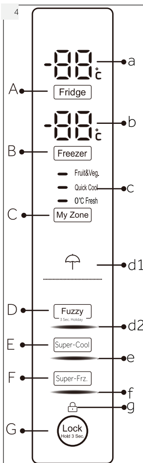
Bedienblende (Abb. 4)
