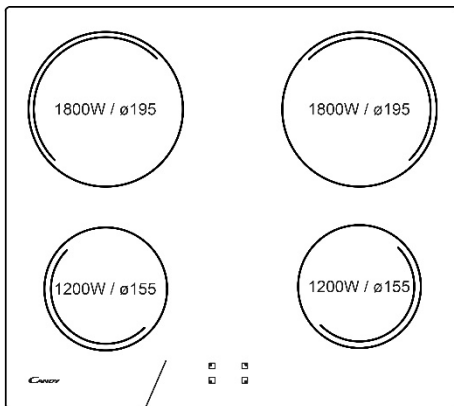
(Versione 2) Figura 3 Superficie in vetroceramica
