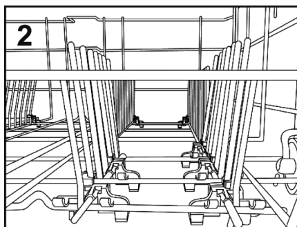
Alsó kosár (2. ábra)
